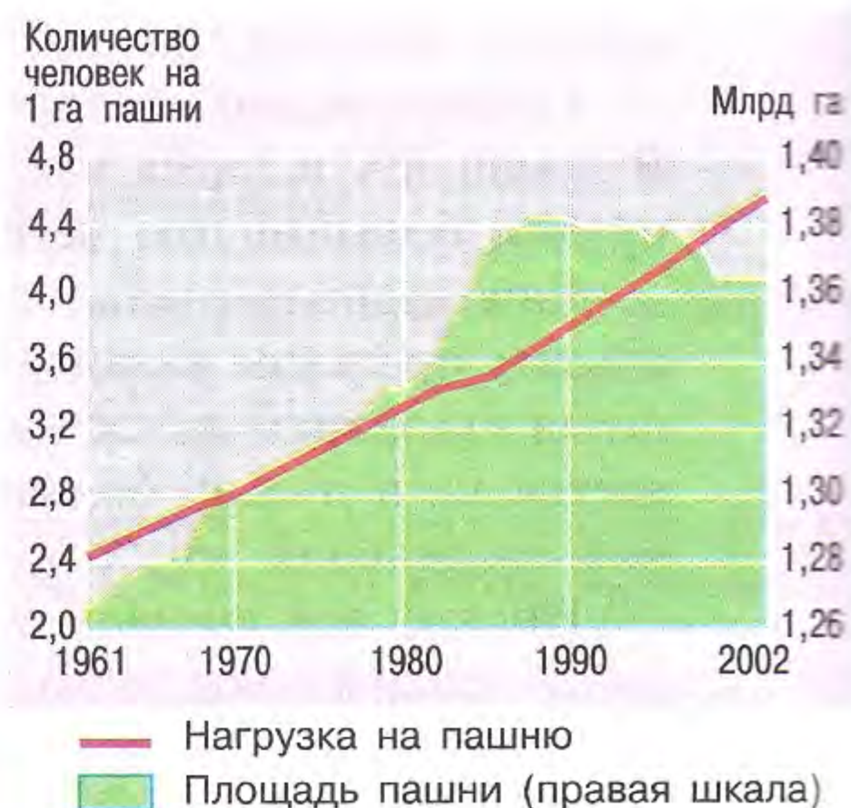
Рис. 90. Рост нагрузки на пашню
