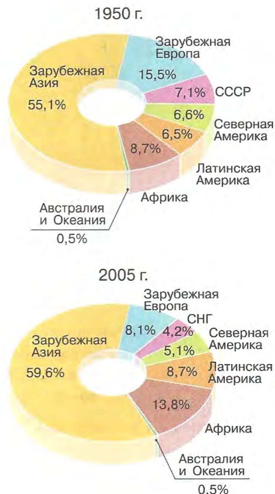
Рис. 20. Динамика численности населения по крупным регионам мира
